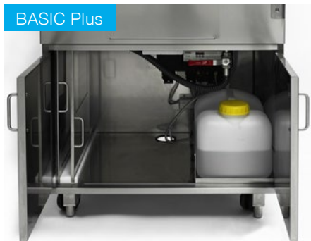
Unterbau mit Flügeltüren, Aufnahmefähigkeit von Wassertank und Pumpe
